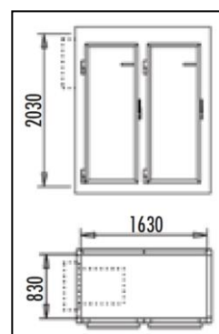
MONOBLOCCO CONDENSAZIONE AD ARIA
